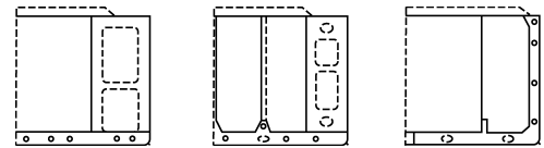
그림 2 Chemical Tanker 'ESP'의 중앙횡단면 예
